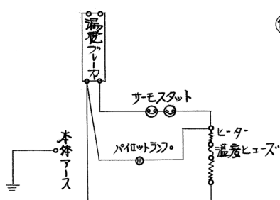
電気回路図
