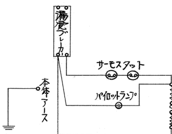
電気回路図
