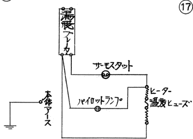
変換回路図
