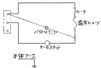
電気回路図
