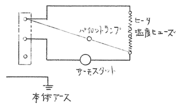
電気回路図
