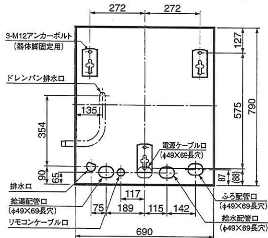
配管、アンカーボルト位置: 上面透視図 [CS-S550TUB-BL]
