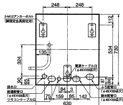
配管、アンカーボルト位置:上面透視図 [CS-S370TB-BL, CS-S460TB-BL]
