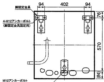
脚固定金具使用時:上面透視図 [CS-S370TB-BL, CS-S460TB-BL]
