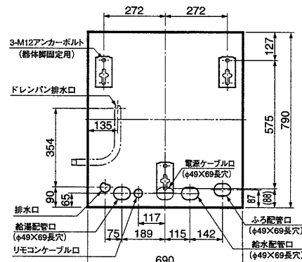
配管、アンカーボルト位置:上面透視図 [CS-S460TBM-BL]
