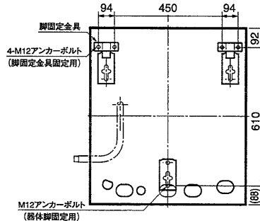
脚固定金具使用時:上面透視図 [CS-S460TBM-BL]
