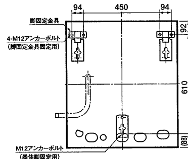
脚固定金具使用時:上面透視図 [CS-S460TBM-BL-H]
