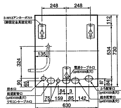
配管、アンカーボルト位置:上面透視図 [CS-S370TB-BL-H、CS-S460TB-BL-H]
