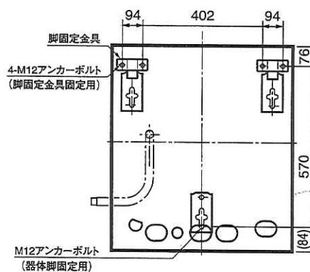
脚固定金具使用時: 上面透視図 [CS-S460TUB-BL]
