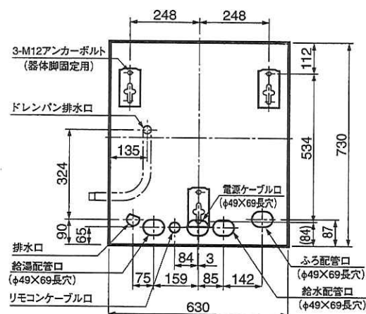
配管、アンカーボルト位置: 上面透視図 [CS-S460TUB-BL]
