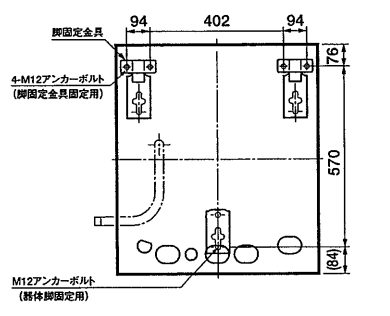
脚固定金具使用時:上面透視図 [CS-S370TB-BL-H、CS-S460TB-BL-H]
