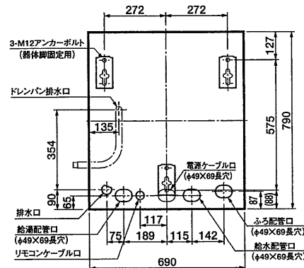
配管、アンカーボルト位置:上面透視図 [CS-S460TBM-BL-H]
